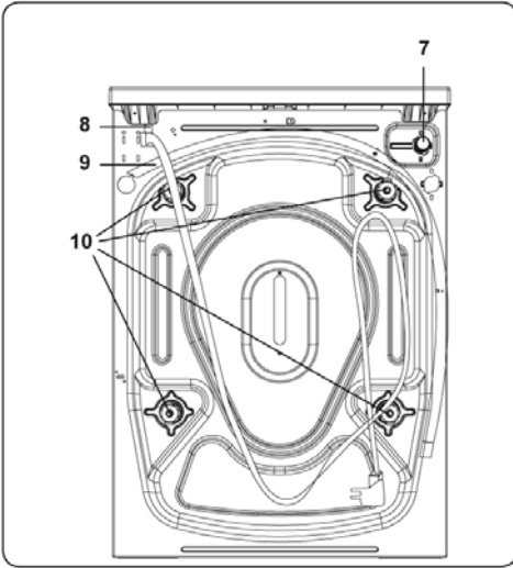
גב המכונה
